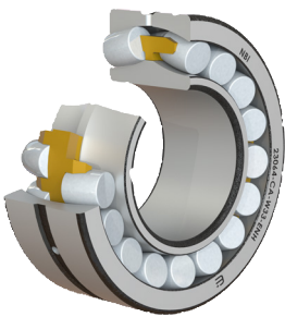
SRB (Rodamiento de rodillos esféricos)
